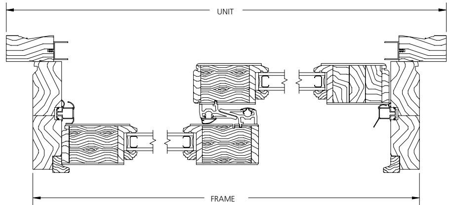
HORIZONTAL SECTION 4 9/16" JAMB
