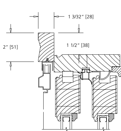
BRICKMOULD
