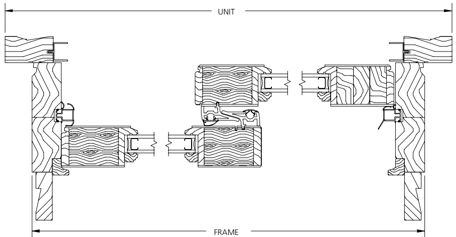
HORIZONTAL SECTION 6 9/16" JAMB
